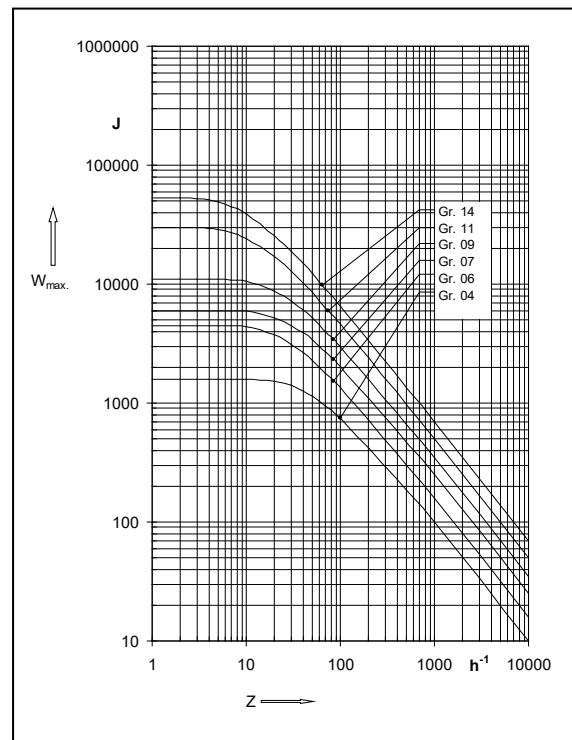
Abb. 24/1: Höchst-Schaltarbeit W_{max} pro Schaltung in Abhängigkeit von der stündlichen Schaltzahl Z (Werte gelten für n=1000\text{min}^{-1} )
