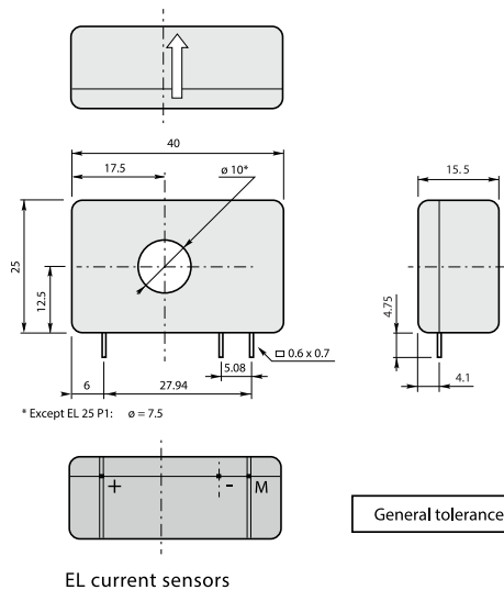
EL current sensors
